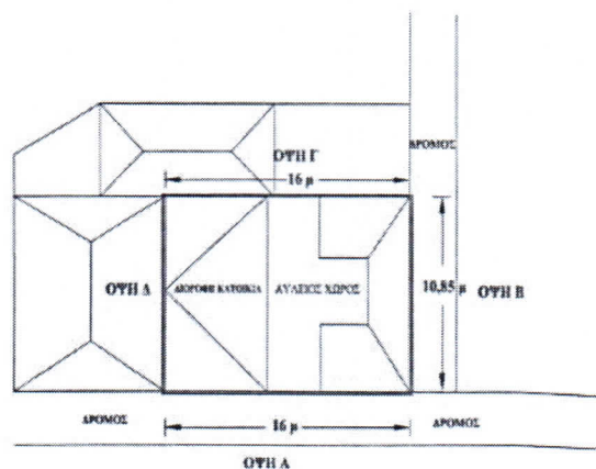
Φωτ 2 Σκαρίφημα αυτοψίας αρμόδιου μηχανικού Δήμου Αριστοτέλη.
