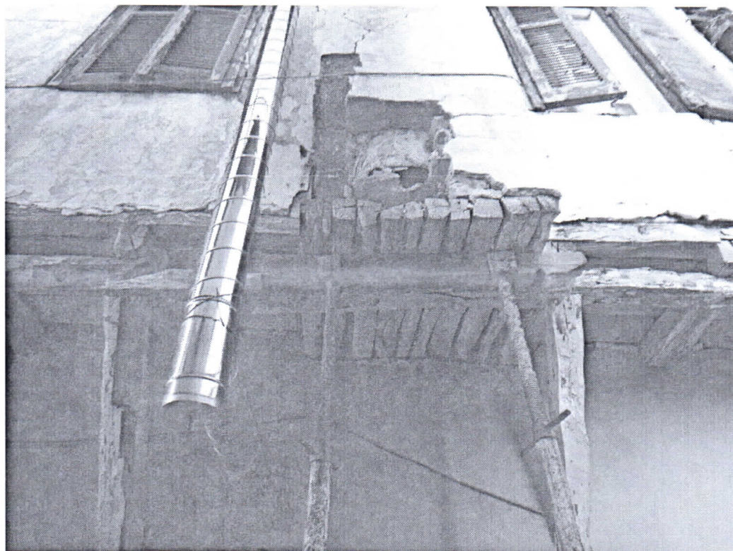
Φωτ 8 Λεπτομέρεια παθολογίας καπνοδόχου
