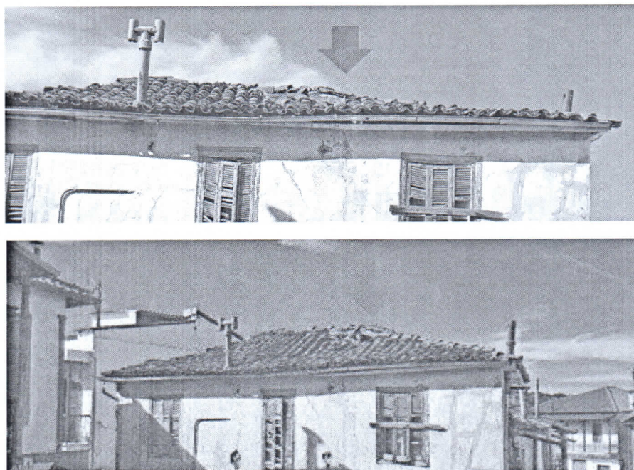
Φωτ 7-8 Λεπτομέρειες στέγης, όπου διακρίνεται το τμήμα της στέγης που έχει καταπέσει
